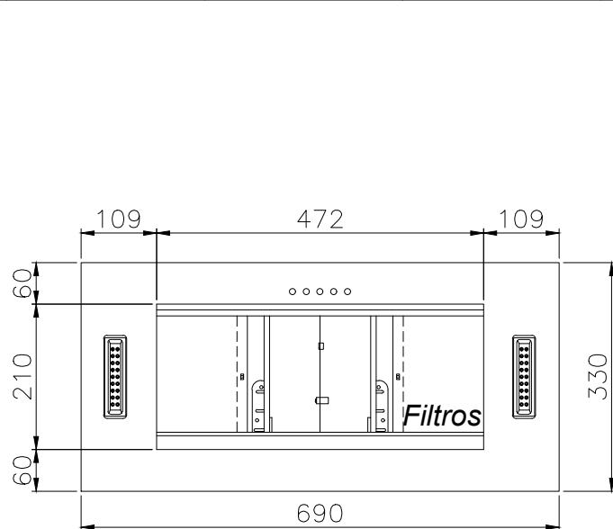
Vista Inferior
