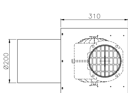
Vista Inferior
