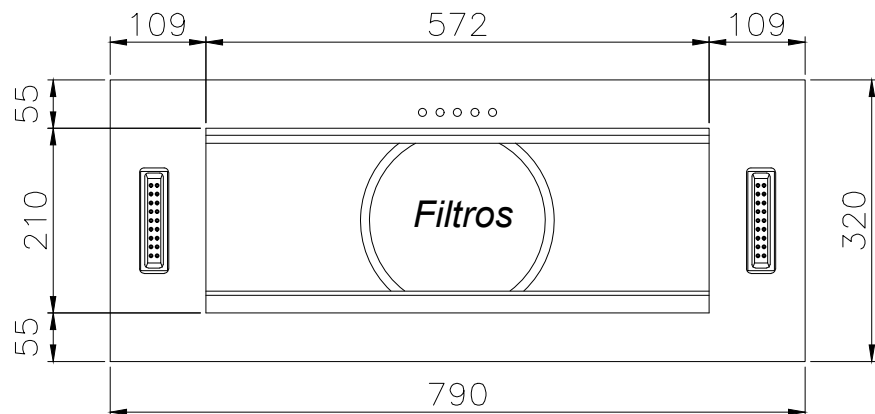
Vista Inferior
