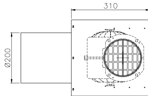
Vista Inferior
