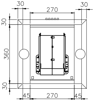
Vista Inferior
