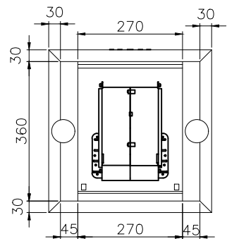
Vista Inferior
